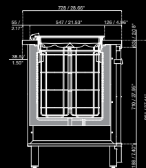
Banco PANORAMA con riserva PANORAMA counter with two levels of gelato tubs Comptoir PANORAMA avec réserve PANORAMA-Treske mit Vorrat Mostrador PANORAMA con reserva
