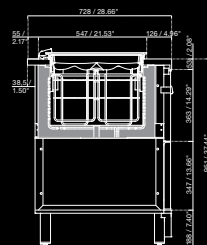
Banco PANORAMA senza riserva PANORAMA counter with one level of gelato tubs Comptoir PANORAMA sans réserve PANORAMA-Treske ohne Vorrat Mostrador PANORAMA sin reserva
