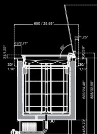
Vasca da incasso PANORAMA con riserva PANORAMA built-in tank with two levels of gelato tubs Cuve PANORAMA encastrable avec réserve Einbaus-PANORAMA-Wanne für Gelato/Granita mit Vorrat Cuba PANORAMA empotrada con reserva
