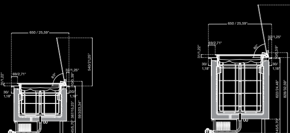
Vasca da incasso PANORAMA senza riserva PANORAMA built-in tank with one level of gelato tubs Cuve PANORAMA encastrable sans réserve Einbaus-PANORAMA-Wanne für Gelato/Granita ohne Vorrat Cuba PANORAMA empotrada sin reserva
